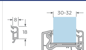
Con junquillo 20-22 Sliding Acristalamiento 30-32
