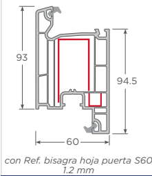
con Ref. bisagra hoja puerta S60 1.2 mm Hoja Puerta Interior
