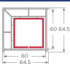
Esquinero 90° 60mm S60
