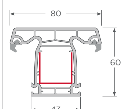
Poste T S60
