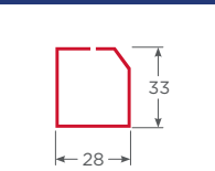
Ref. Box Marco Fijo Inclinado S60 1.2mm - TC PL-S60-TC-BMF-12
